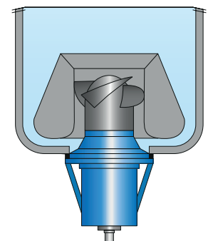
Agitador compacto de fondo de cuba
