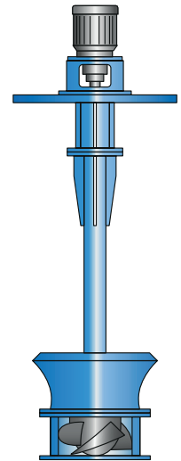
Agitador línea de eje
