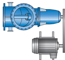
Accionamiento por correas trapezoidales, motor sobre guías
