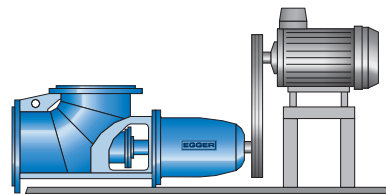
Accionamiento por correas trapezoidales
