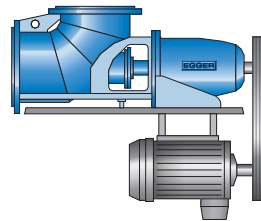
Accionamiento por correas trapezoidales, motor suspendido
